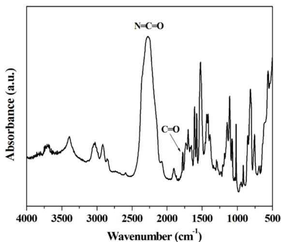
Figure S2. FTIR spectrum of MDI.
